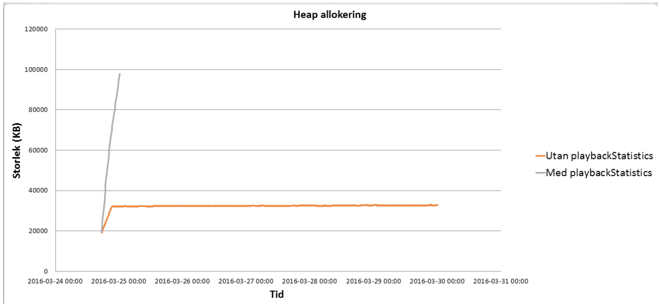
Illustration 15: Minnesallokeringen med samt utan funktionen som orsakade minnesläckan.
